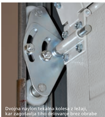
Okovje vrat vključno s torzijskimi vzmetmi je vroče pocinkano Galvanized door carriages and torsion springs
